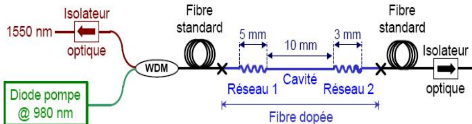
Figure I.16 : Présentation des lasers à réflecteurs de Bragg répartis.
