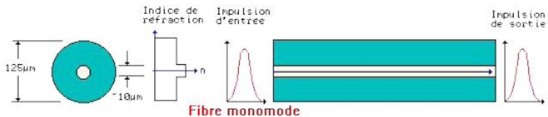
Figure I.11 : Fibre optique Monomode.
